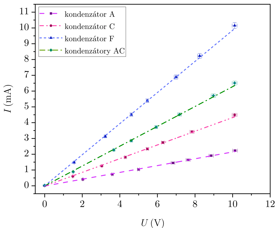
Graf 1: Závislost proudu I na napětí U při měření kapacity C kuličkové kapacitní dekády v různých konfiguracích
